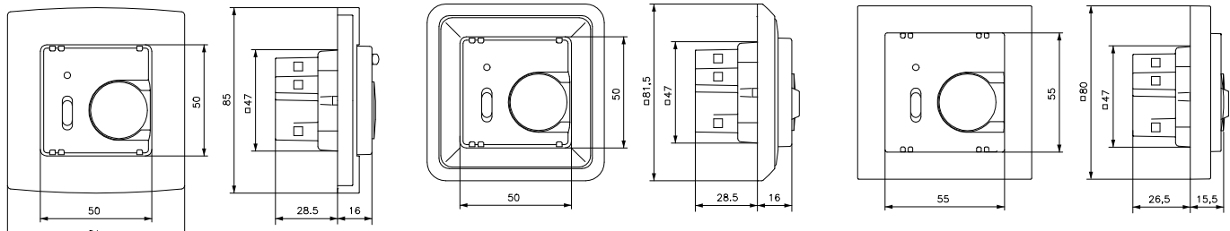
Régulateur 50x50 mm avec cadre standard Регулятор 50 x 50 mm стандартной рамкой
